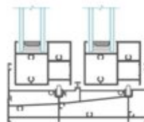
高轨设计 High-rail design 提升密封，防水性能
